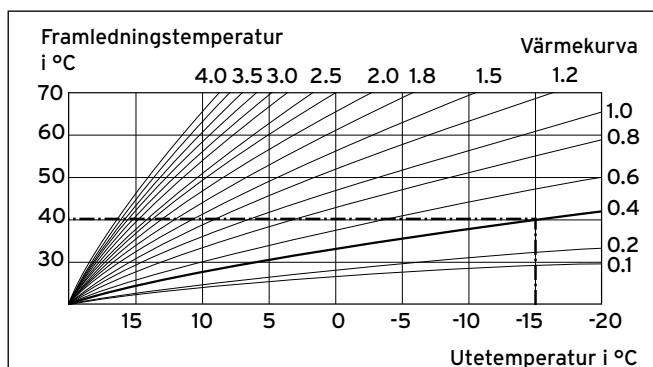
10.1 Diagram värmekurvor
