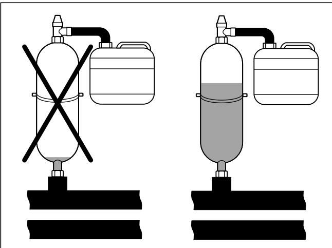
6.1 Nivån i expansionskärlet för brine
