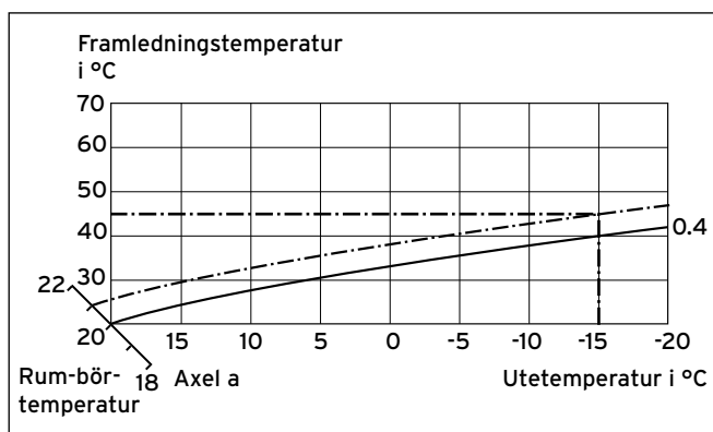
10.2 Parallellförskjutning av värmekurvan
