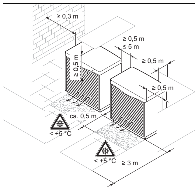
Avstånd som skall iakttas vid två luft-brine-enheter
