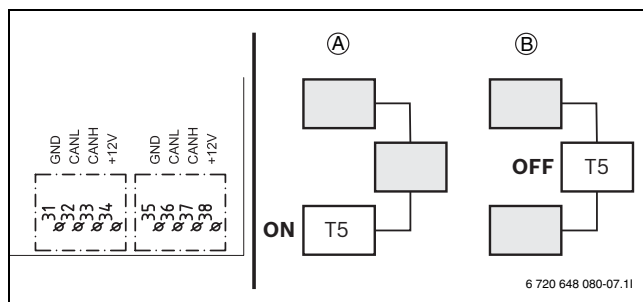
Bild 4 Terminering CANbus LCD
