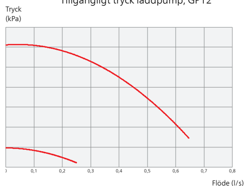
Tillgängligt tryck laddpump, GP12
