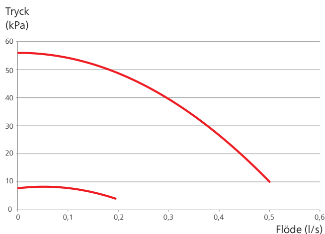
Tillgängligt tryck cirkulationspump, GP1
