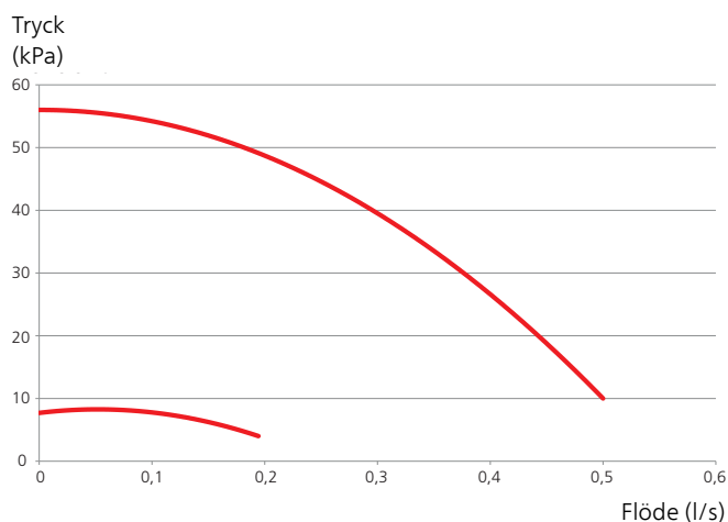
Tillgängligt tryck laddpump, GP12
