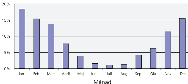
% av årsförbrukningen Bergvärmepumpens energifördelning fördelat över året
