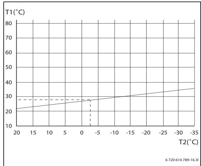
Bild 22 Golv
