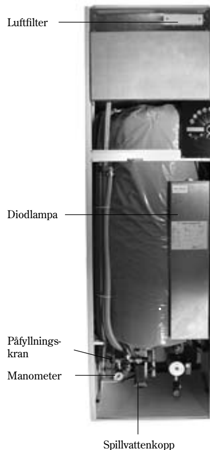
IVT 490
