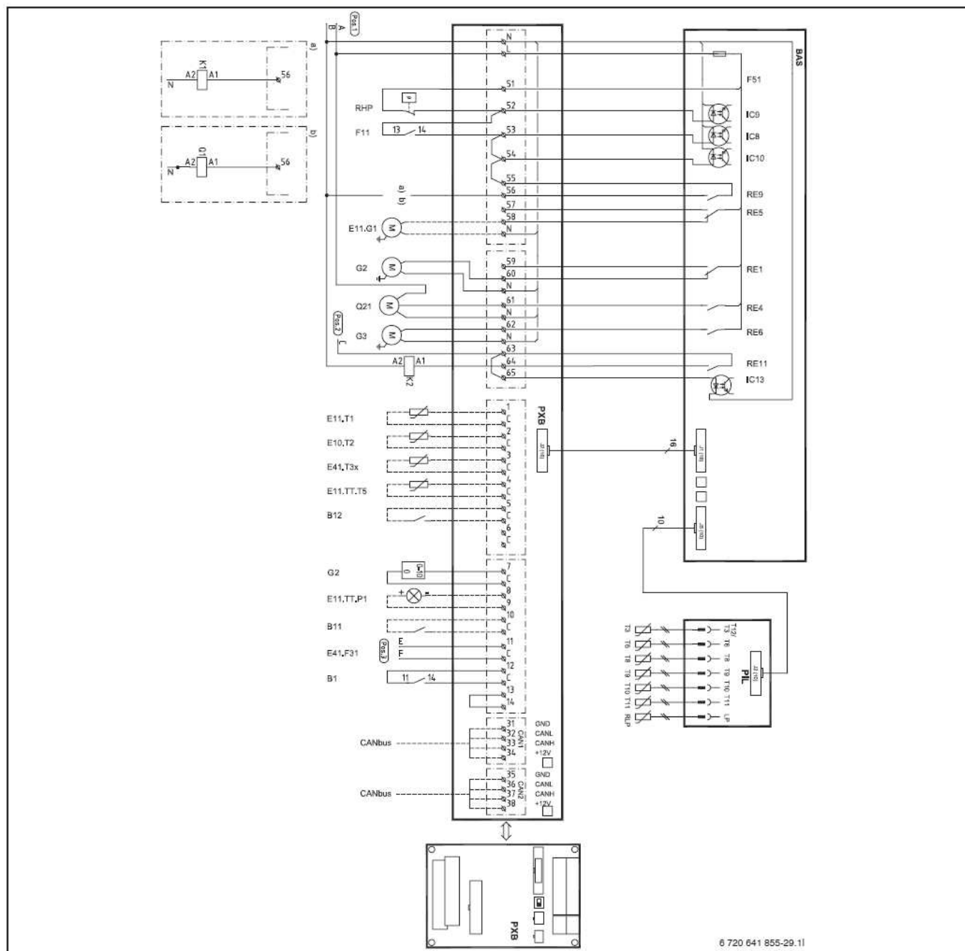
Bild 47 Komplett elschema anslutningar
