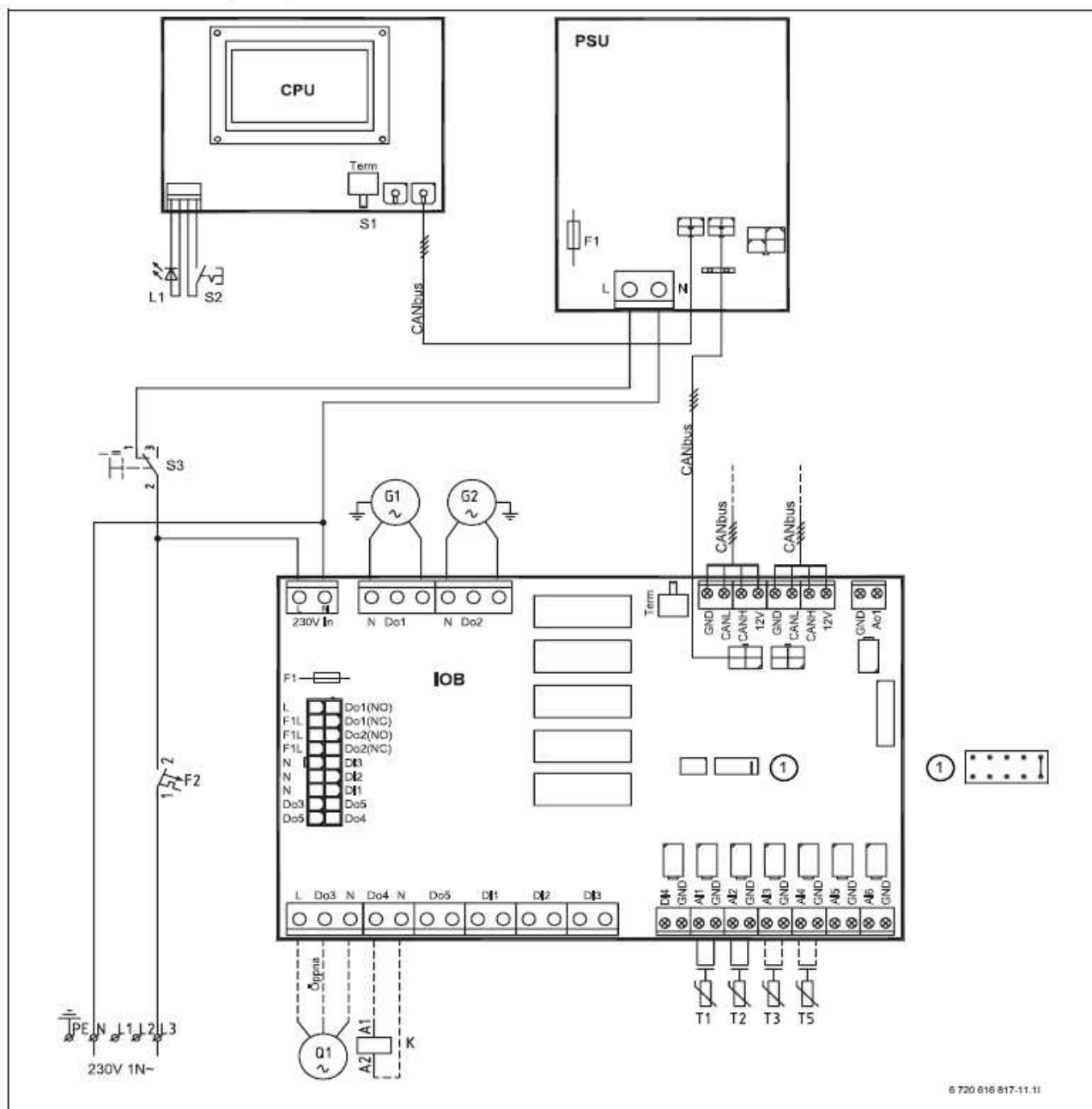
Bild 57 Kretsschema styrskåp
