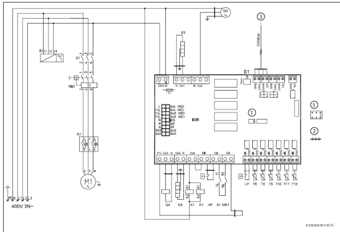
Bild 48 Elschema Air 50-90
