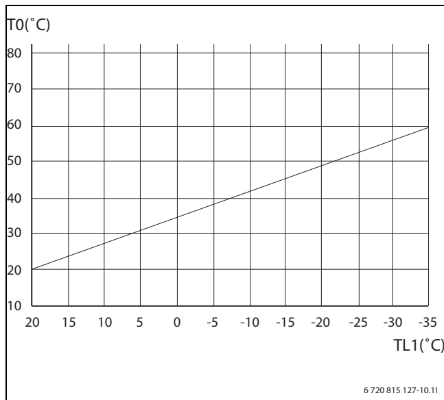
Bild 2 Radiatorsystem
