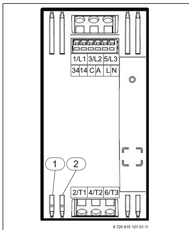
Bild 5 Mjukstart
