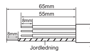
Kommunikationskabel
