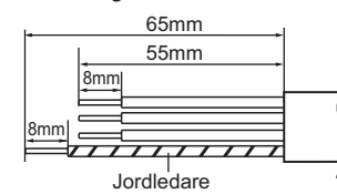
Anslutningskabel
