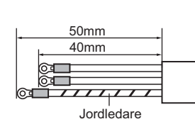
Strömförsörjningskabel
