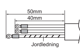
Strømkabel
