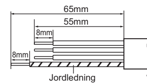
Tilkoblingskabel
