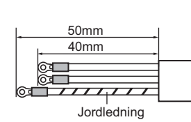
Strømforsyningskabel
