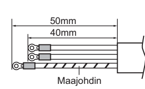
Virransyöttökaapeli
