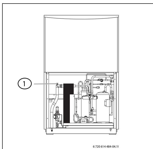
Bild 28 Värmepump
