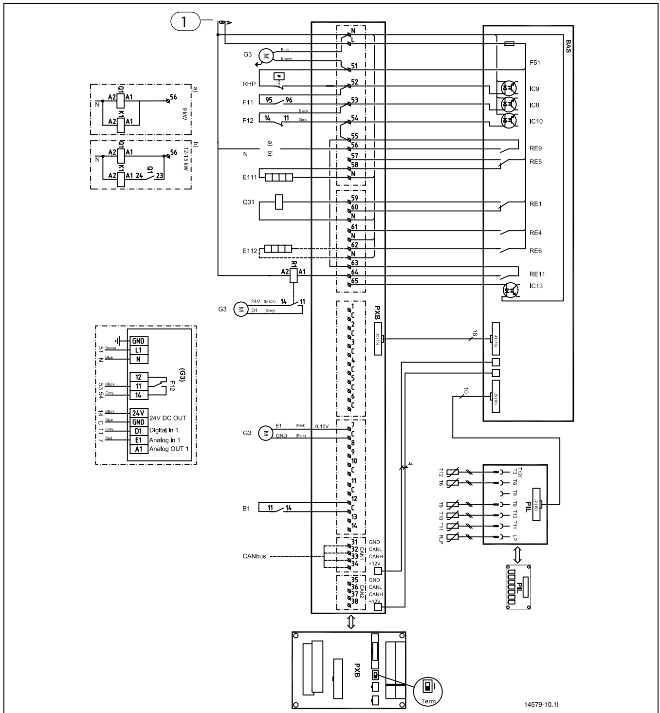
Bild 32 Anslutningar värmepump
