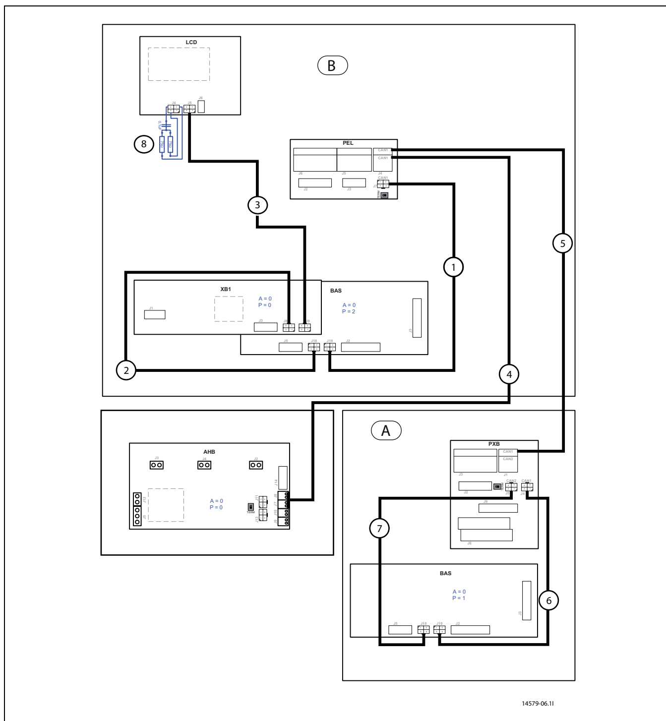
Bild 4 CANbus kopplingsschema värmepump, styrskåp och tillskott
