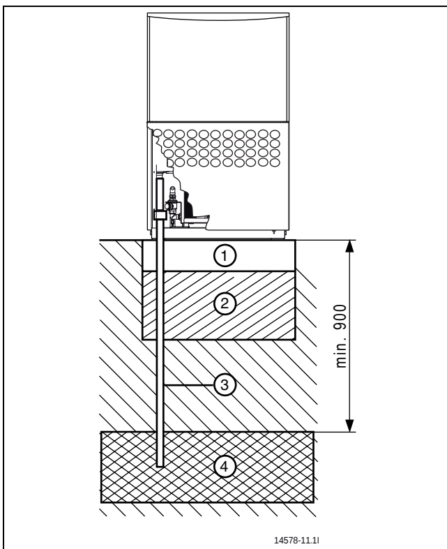
Bild 23 Avrinning kondens
