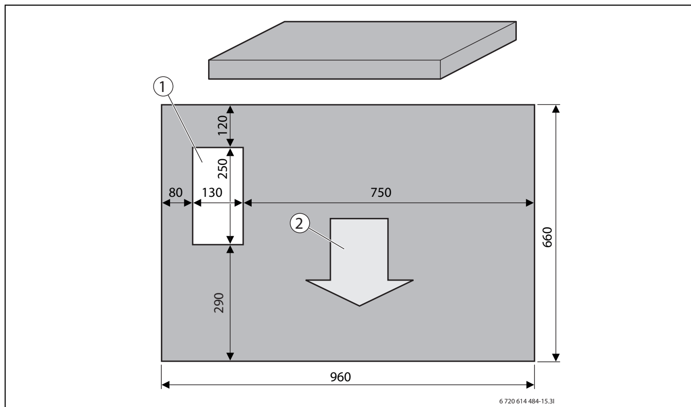
Bild 18 Mått för fundament
