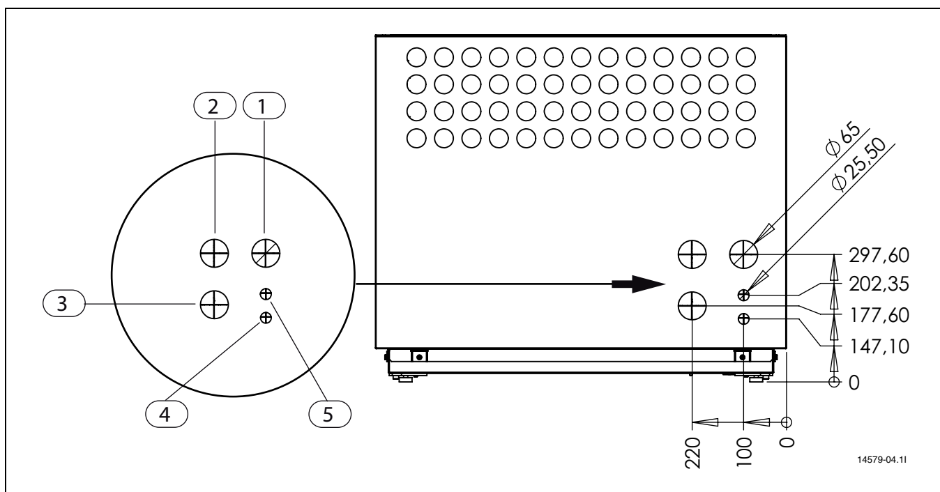
Bild 17 Måttsättningar och anslutningar värmepump
