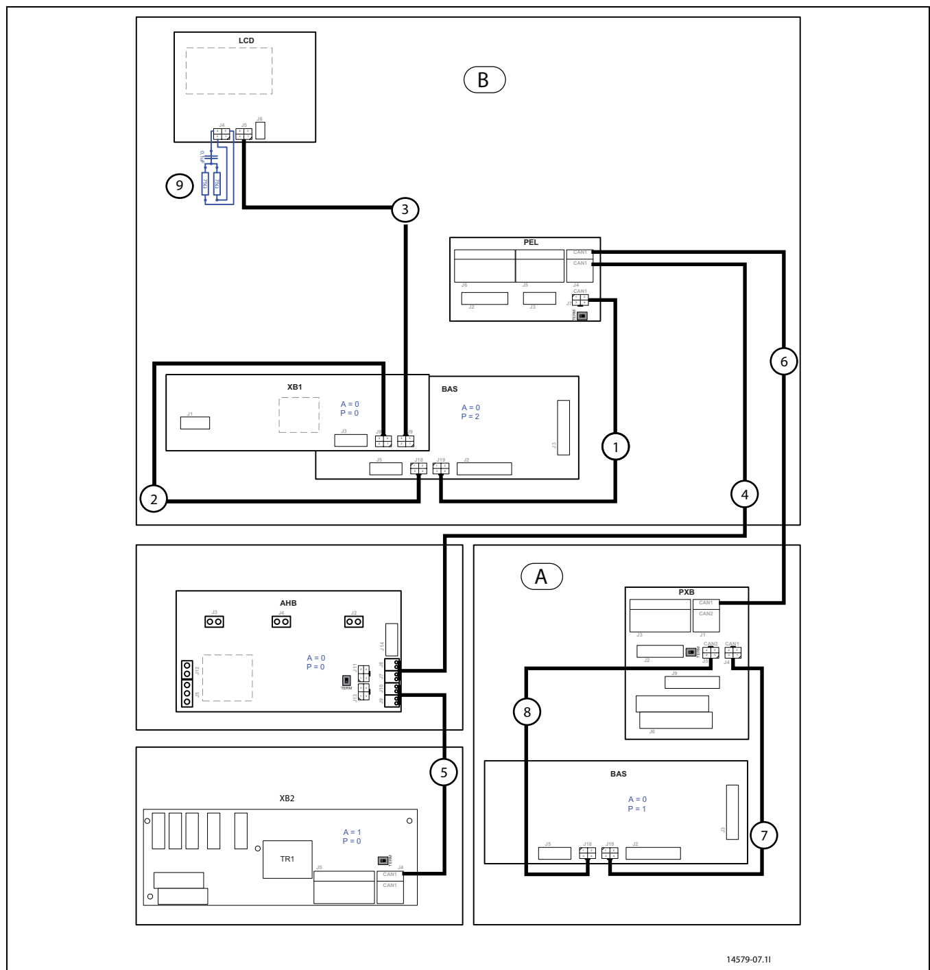
Bild 5 CANbus kopplingsschema värmepump, styrschåp, tillskott och tillval
