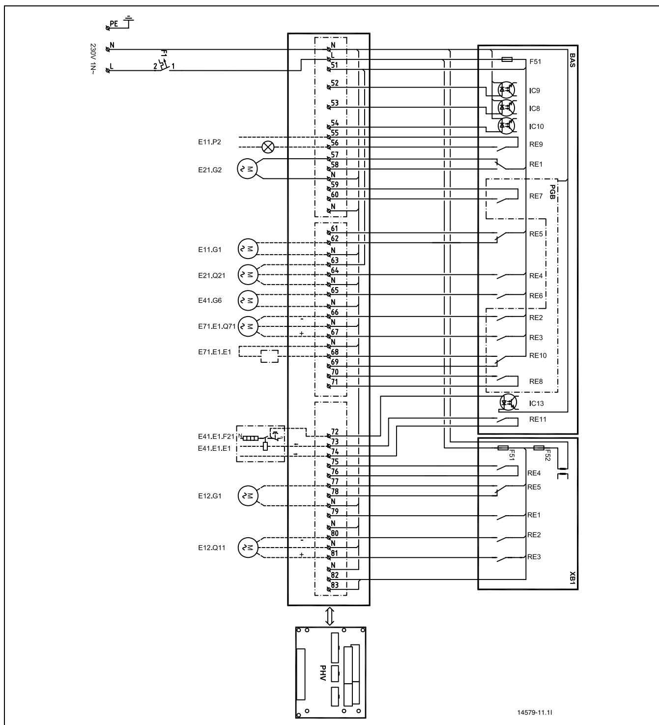
Bild 34 Anslutningar styrsåp
