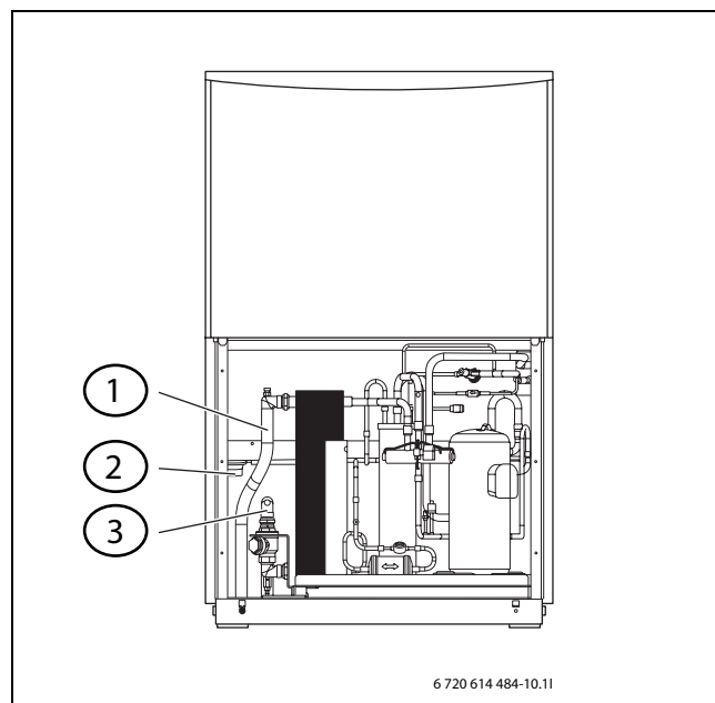
Bild 16 Anslutningar värmepump
