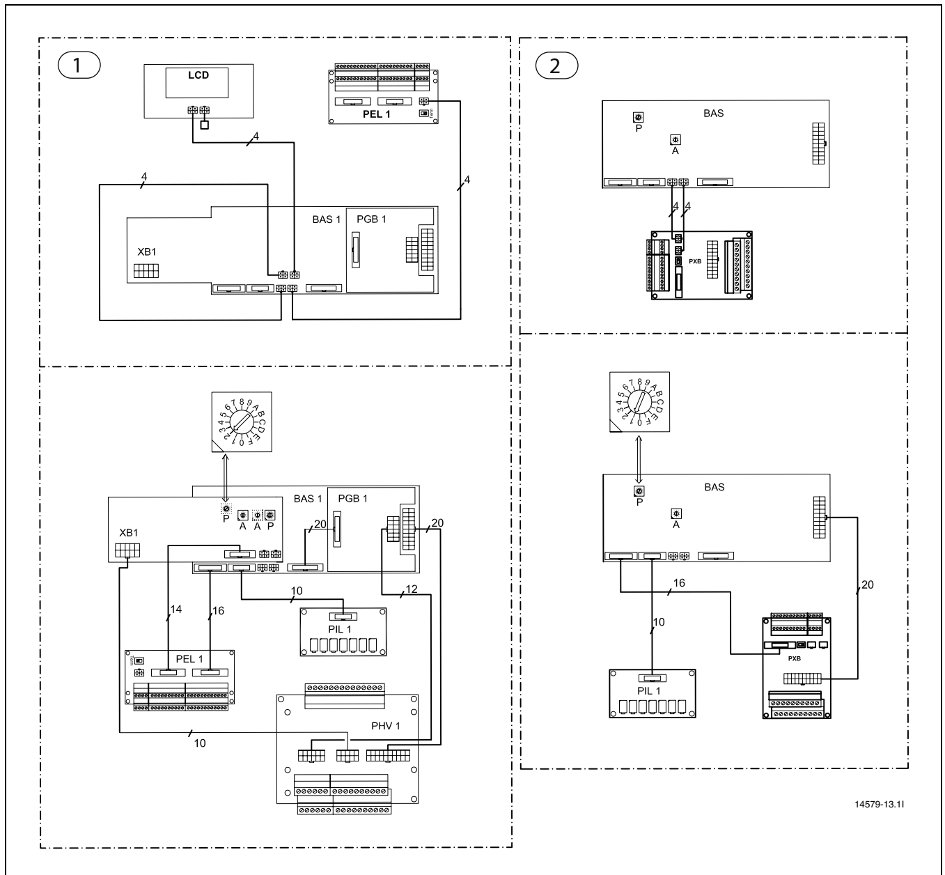
Bild 30 Kretskort styrsåp och värmepump
