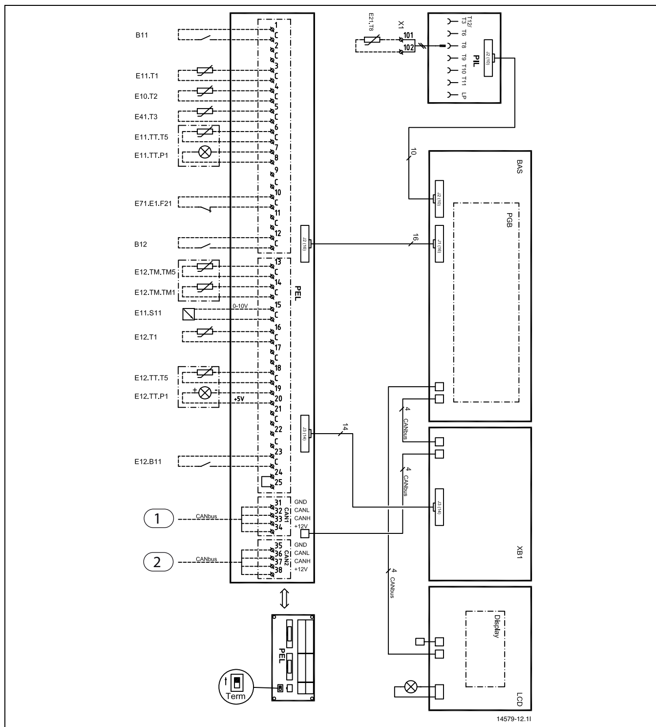
Bild 33 Elschema styrsåp
