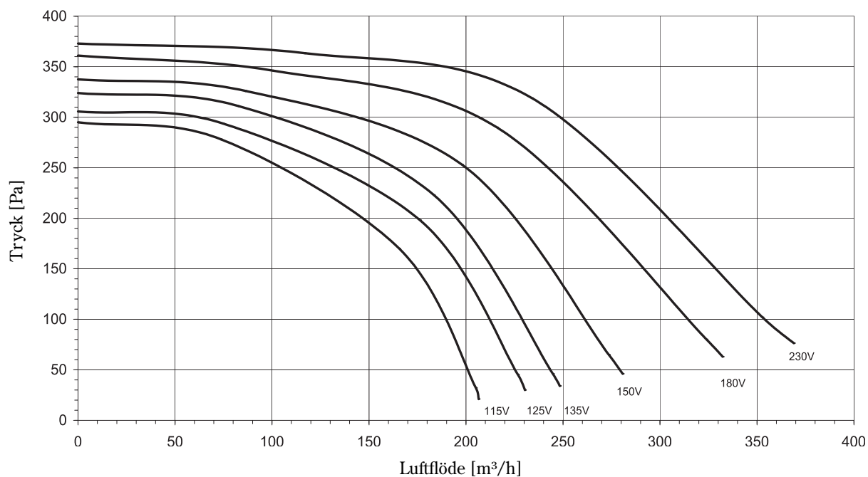
Tryck/Luftflöde diagram
