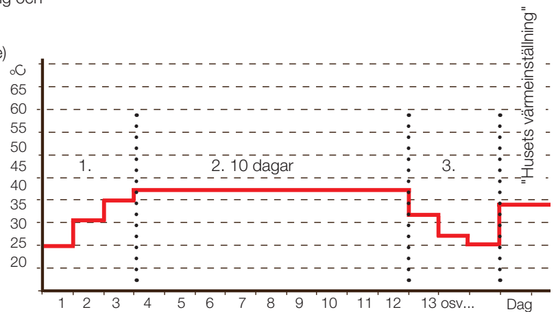
Exempel för Mode 2 med "Golvfunktion temp°C 37 °C.
