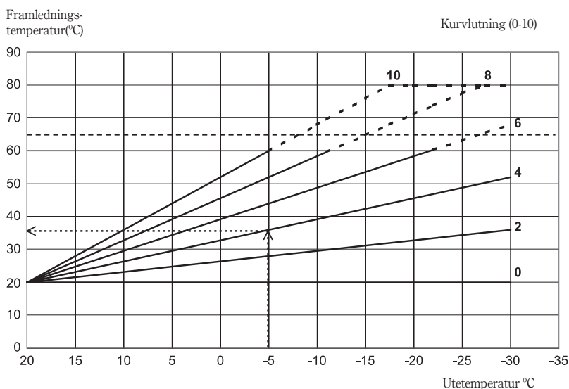
Värmekurvan
