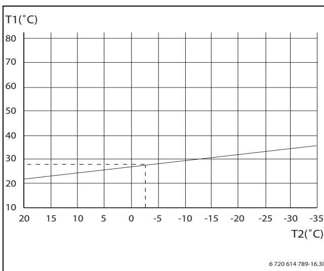
Bild 21 Golv
