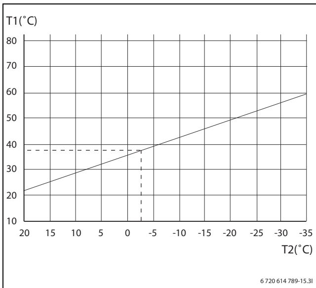
Bild 20 Radiator
