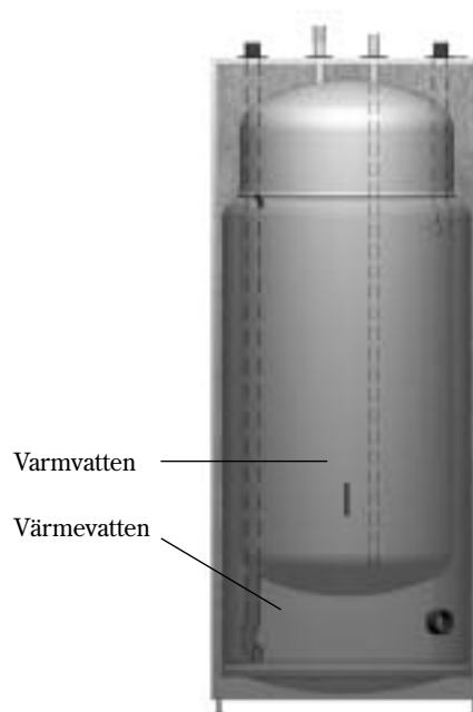
Dubbelmantlad varmvattenberedare
