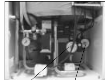
Cirkulationspump för värmesystemet (615 VP-modul)
