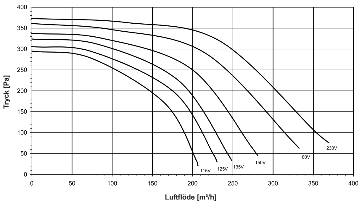
Diagram Tryck/Luftflöde
