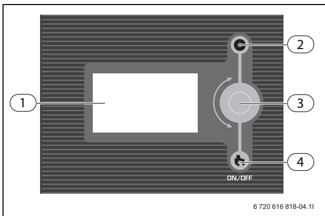
Bild 8 Kontrollpanel CC 160
