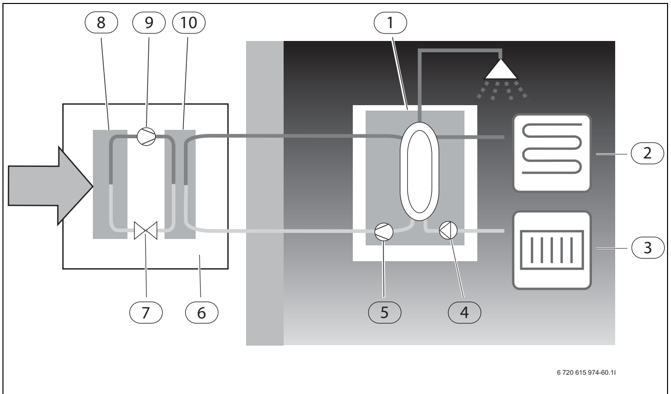
Bild 1 Funktionsbeskrivning EHP AW med CC 160
