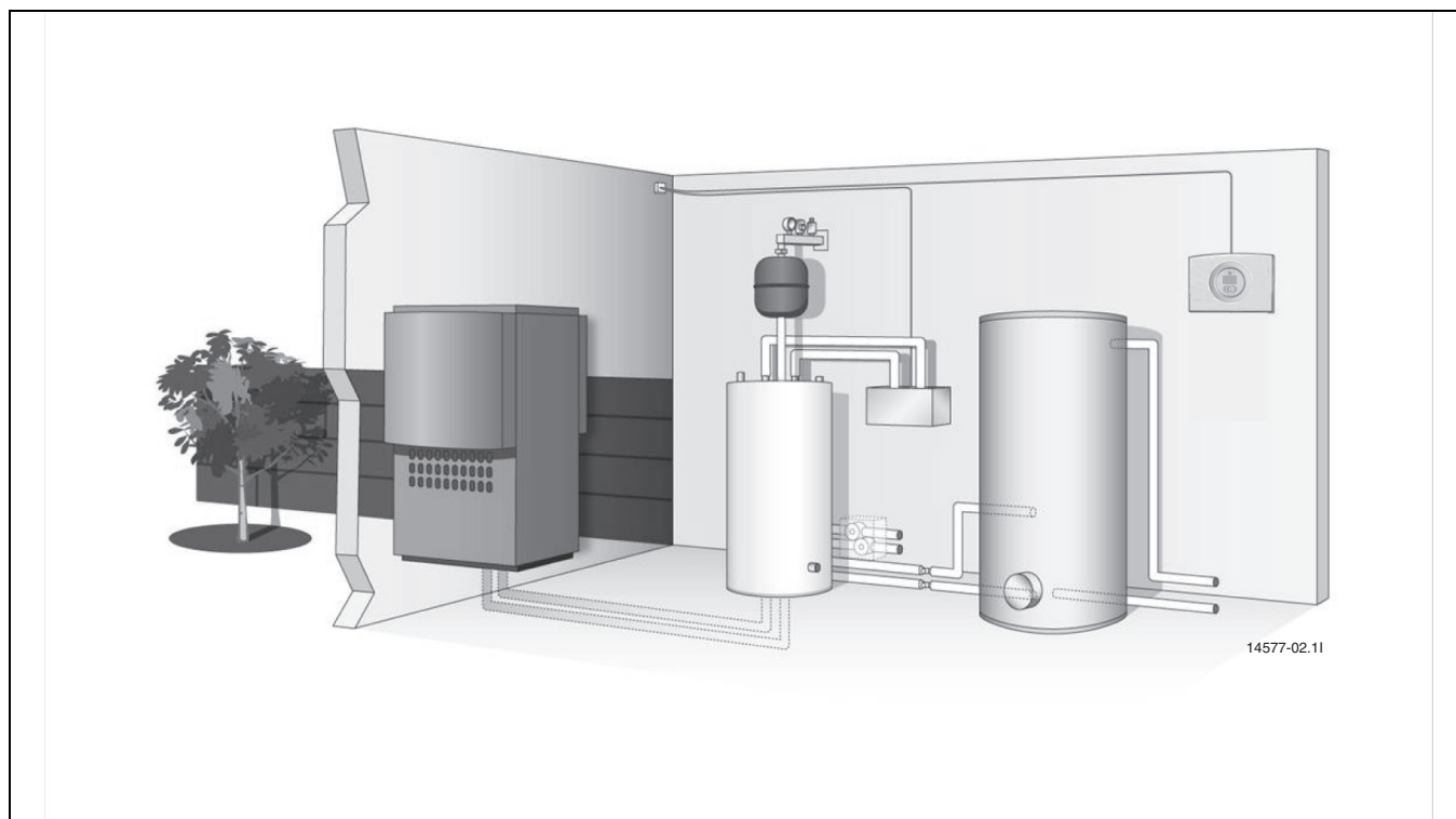
Bild 3 A9–A15 med tillskott
