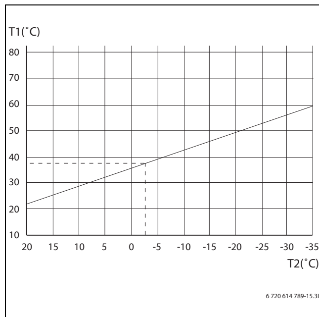
Bild 21 Radiator
