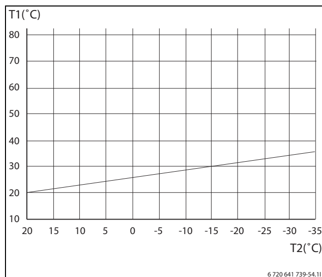
Bild 3 Golvvärme
